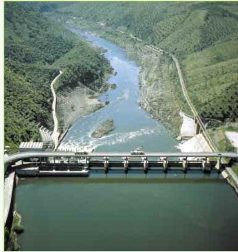
Central Hidroelétrica de Fratel
