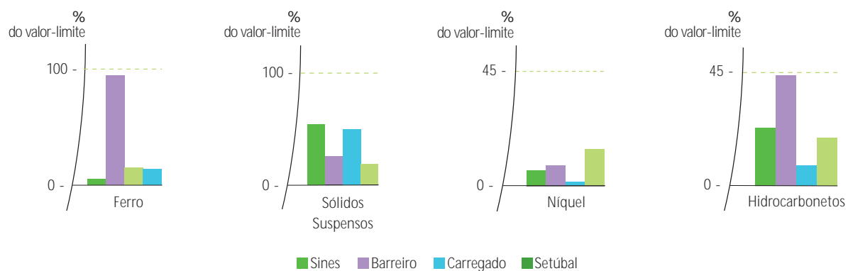
Figura 5A – Ferro, Sólidos Suspensos, Níquel, Hidrocarbonetos
